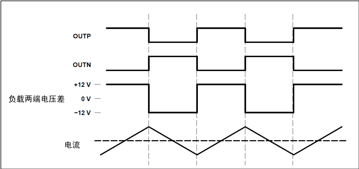
图 1 传统 D 类调制方案
