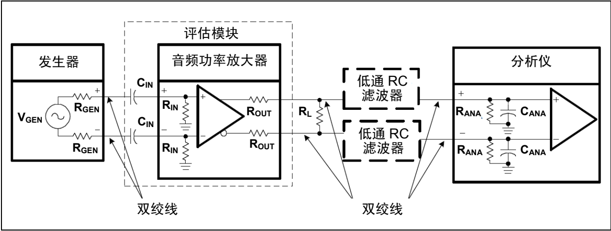
图 6 差分输入、BTL 输出测量电路
