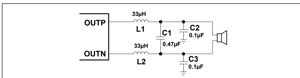
图 3 典型的 LC 输出滤波器，截止频率 27 kHz，扬声器电阻 8 \Omega
