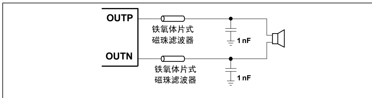
图 4 典型的铁氧体磁珠滤波器
