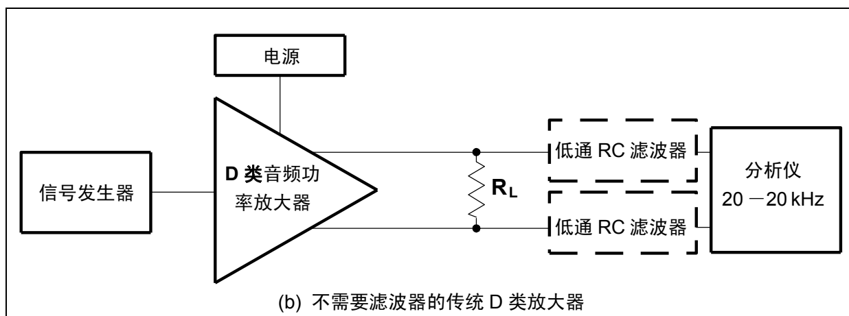
图 5 音频测量系统
