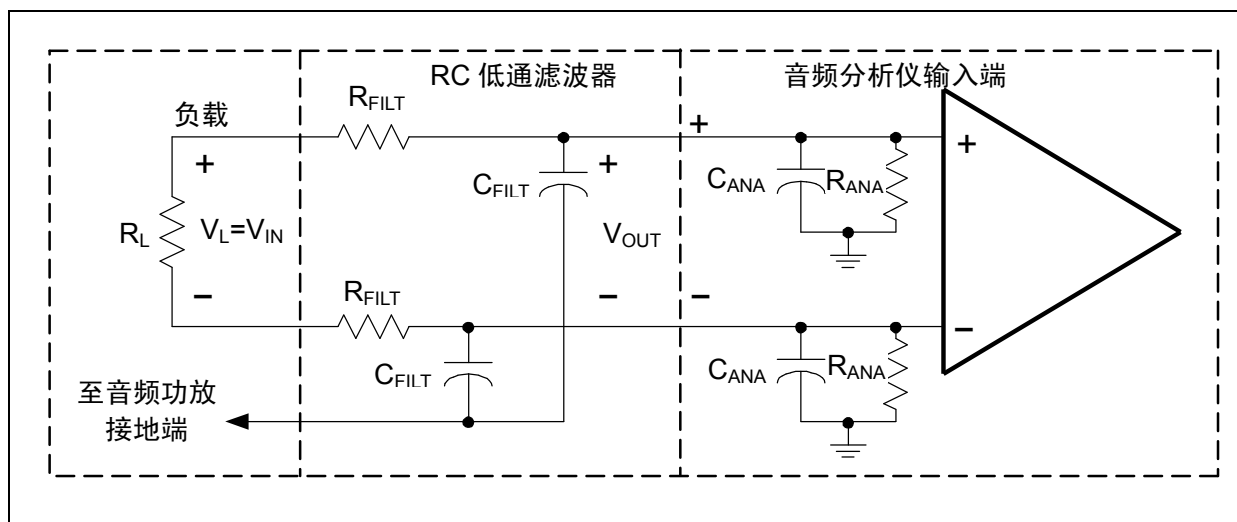
图 7 D 类音频功放测量低通滤波器
