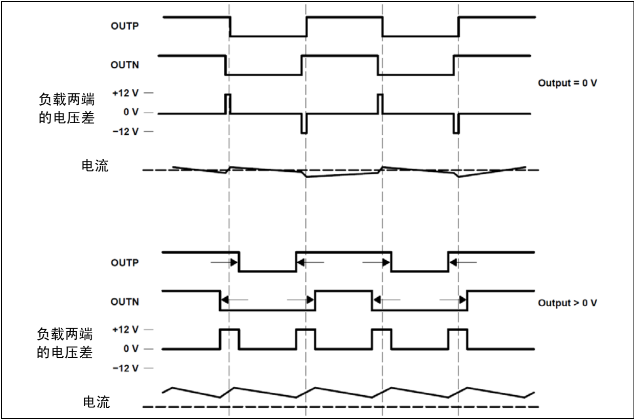
图 2 AX3005 输出电压和电流波形
