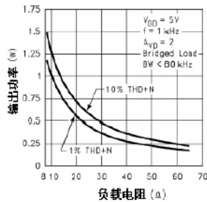
输出功率 vs 负载电阻
