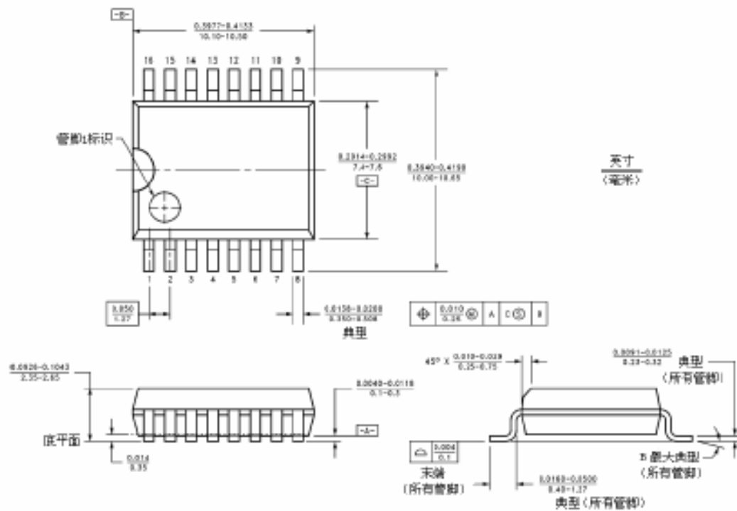
16- 引脚 ( 宽 0.300" ) 模式的 50P 封装, JEDEC
