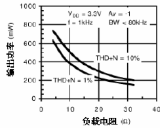
输出功率 vs 负载电阻
