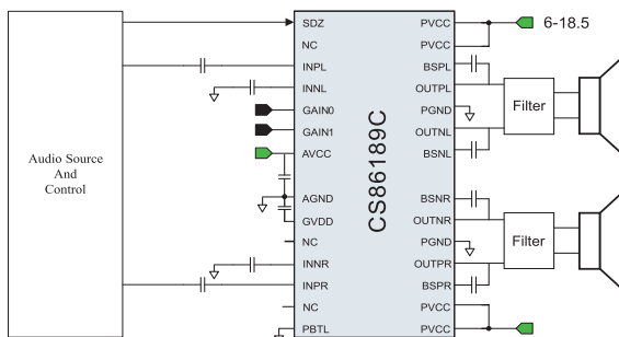
图6 CS86189C单端输入接法
