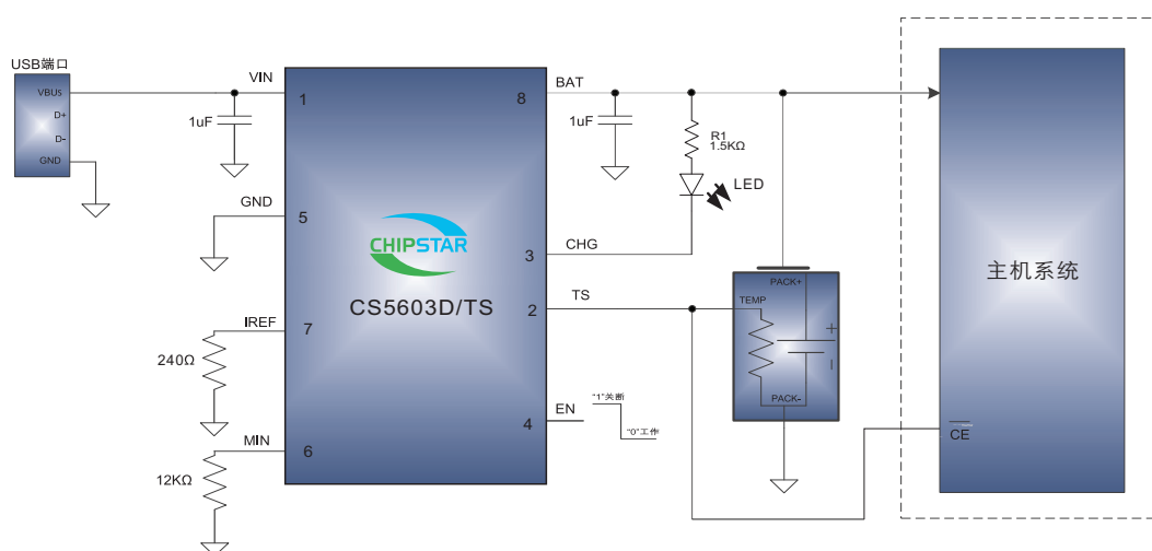
CS5603D/T/S应用电路图
